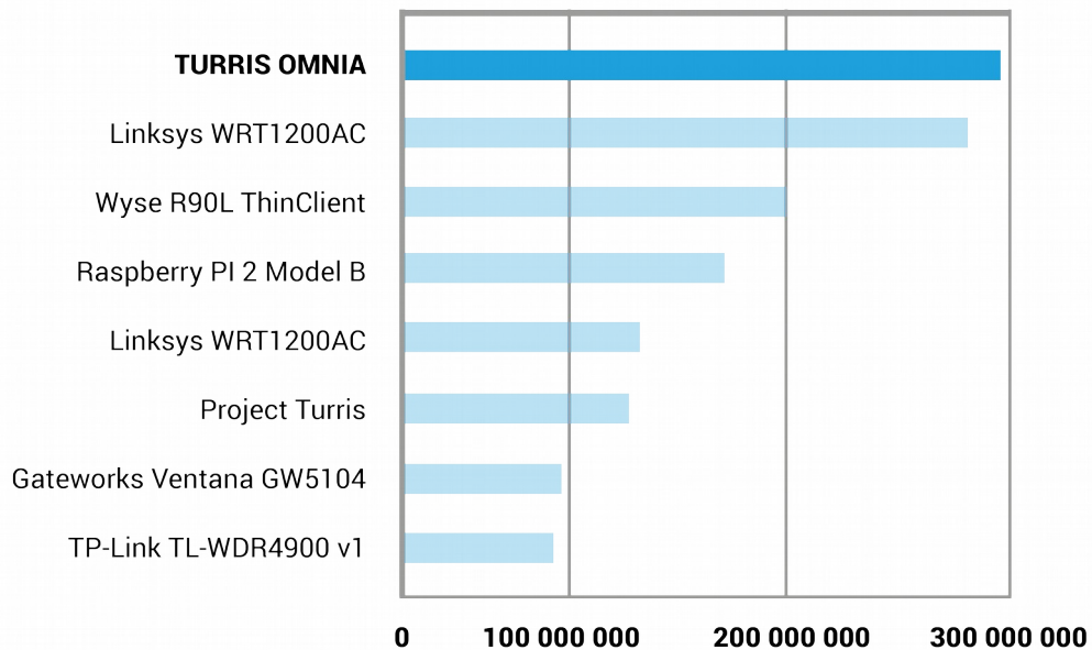
MD5 benchmark
